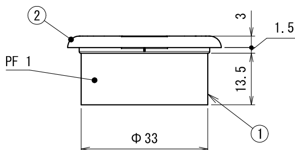
パッキン・ロックナットを外した状態
